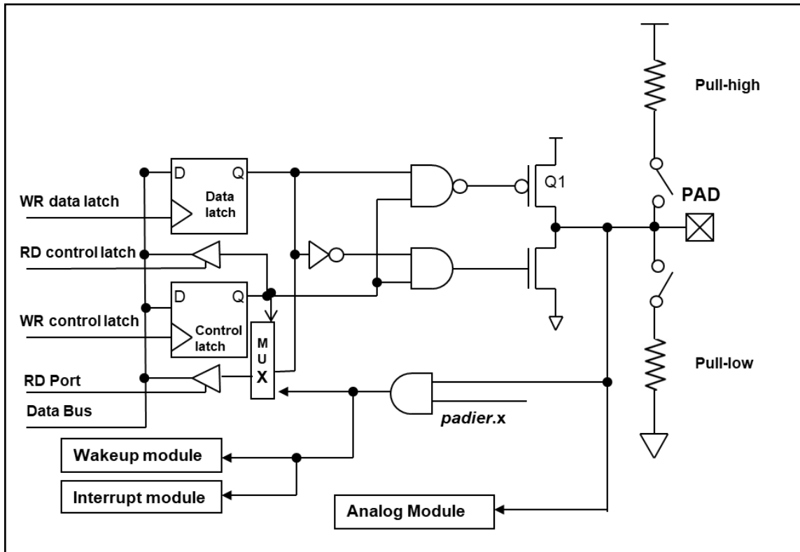
图 18: IO 引脚缓冲区硬件图
