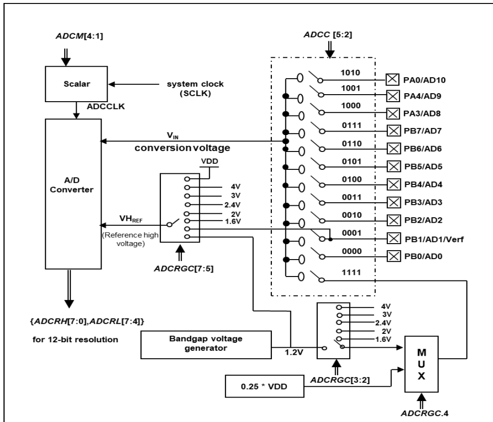
图 19: ADC 模块框图
